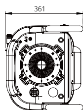
VUE DESSOUS
